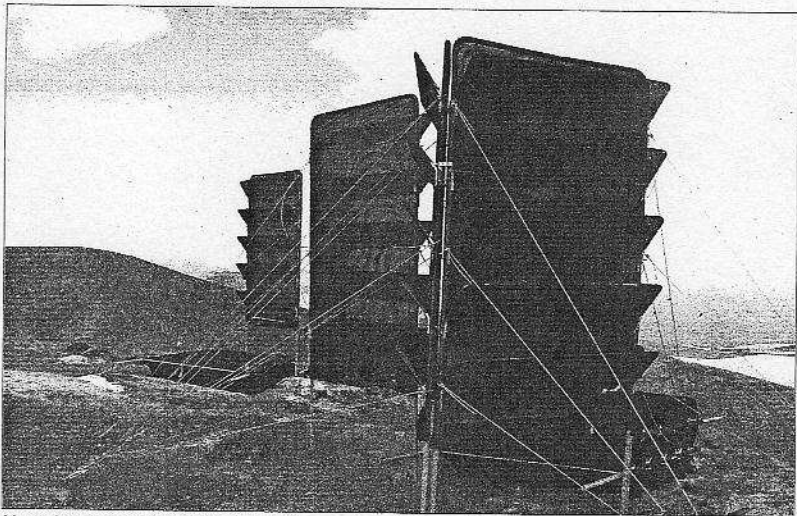
Lluvia horizontal. Las estructuras metálicas condensan la humedad aportada por los vientos alisios.
